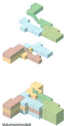
Volumenmodell
